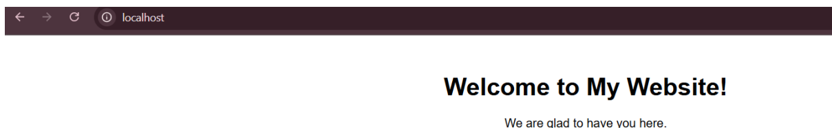
Fig 1.4 chrome output
